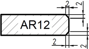
Крайка
